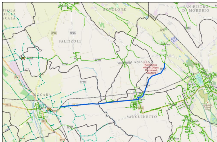
Figura 5-6: Interconnessione Isola-Nogara-Gazzo con Bovolone: collegamento mediano.
