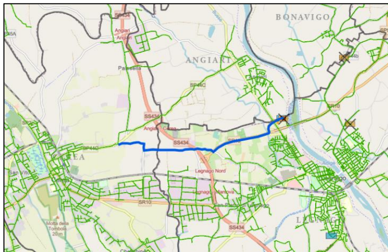
Figura 5-8: Interconnessione tra il sistema di Bovolone e quello di Legnago.
